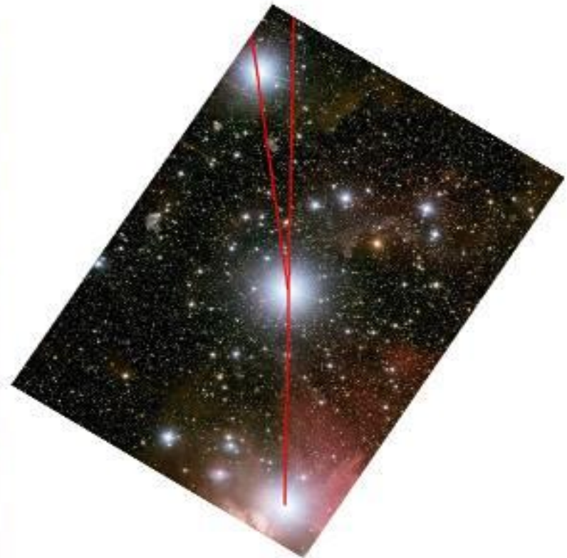
Constelación de Orion
